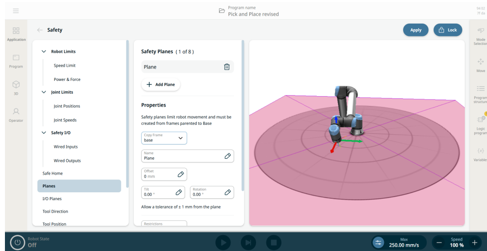
圖 1.5: 顯示安全平面的 PolyScope X 螢幕。
