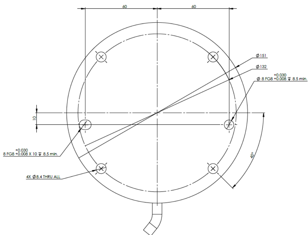
1.1: 機器人底座的底部視圖
